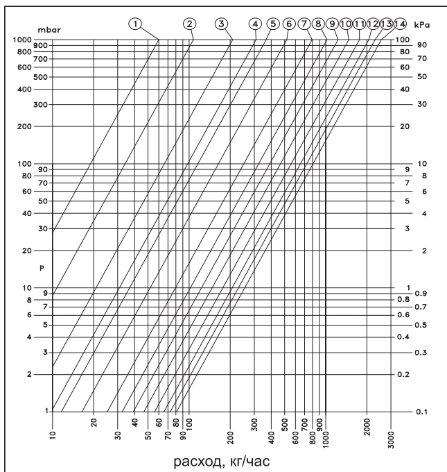
График настройки расхода стопорным винтом
