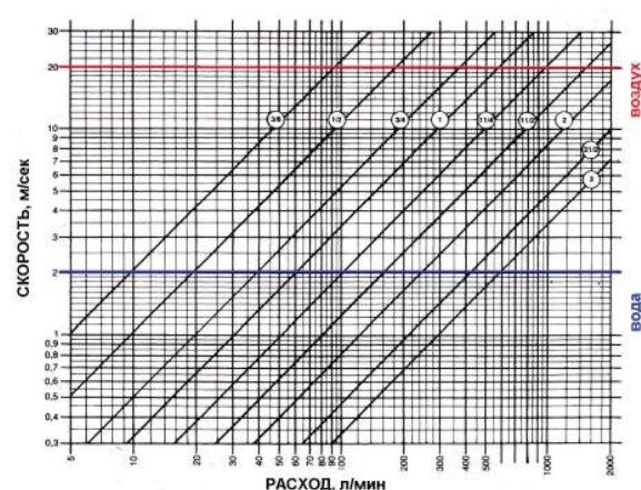
Зависимость скорости от расхода
