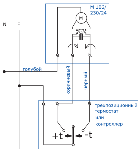
M106 с управлением от трехпозиционного термостата
