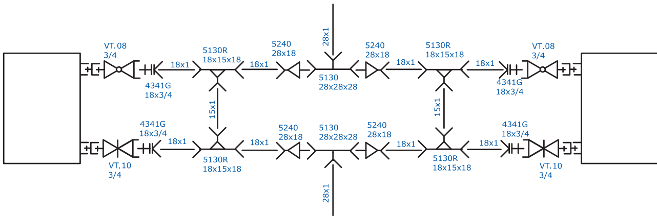
пример монтажной схемы системы на паечных фитингах
