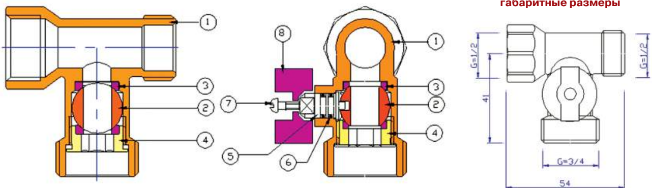
габаритные размеры
