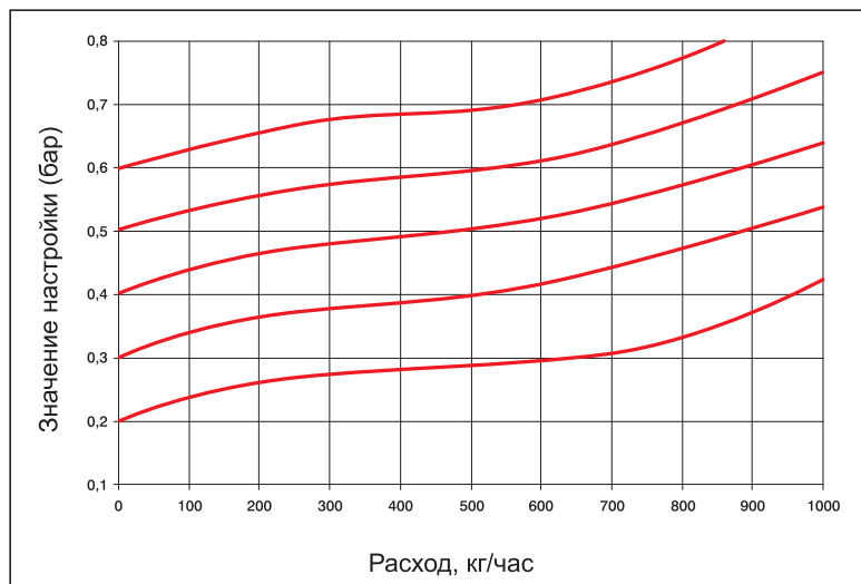
График пропускной способности перепускного клапана
