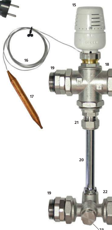
Термостатический модуль
