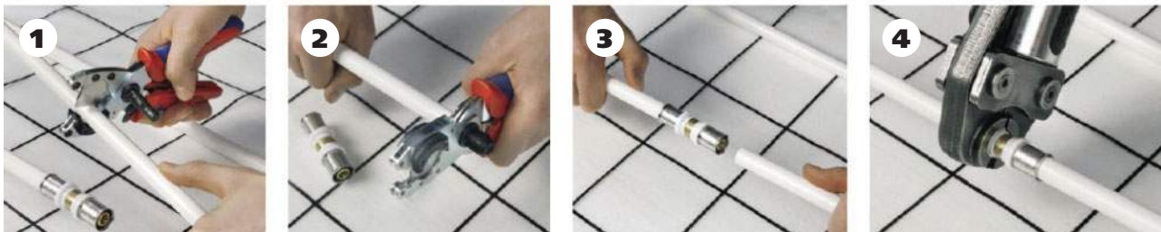
1 Отрезание трубы
