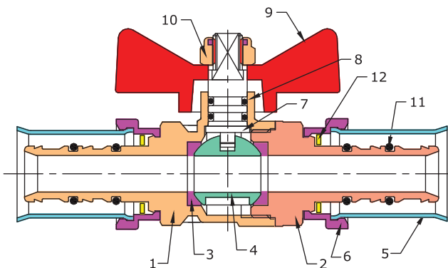
детали крана
